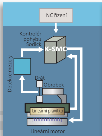
Kontrolér pohybu Sodick
